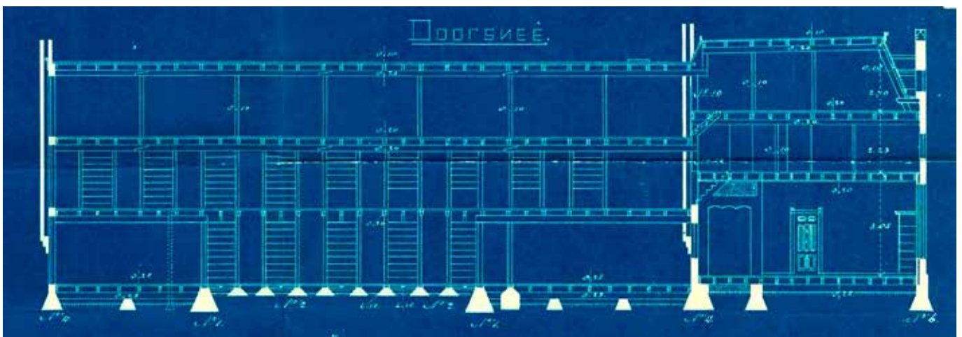
Doorsnede van het gebouw (Bouwarchief Gemeente Hillegom)
